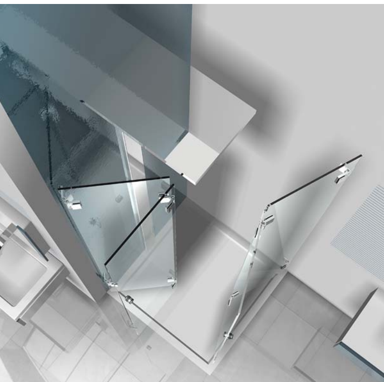
Variante 7 Eckdusche mit 2 Falttüren, Türknauf, Dichtungen und Schwallenschutz Türbreite bis 100 cm
