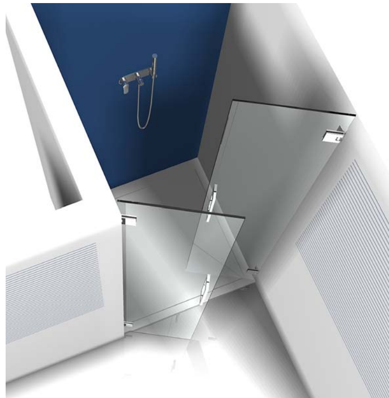
Variante 2 Nischendusche mit 2 Türen, Griffstangen, Dichtungen und Schwallenschutz
