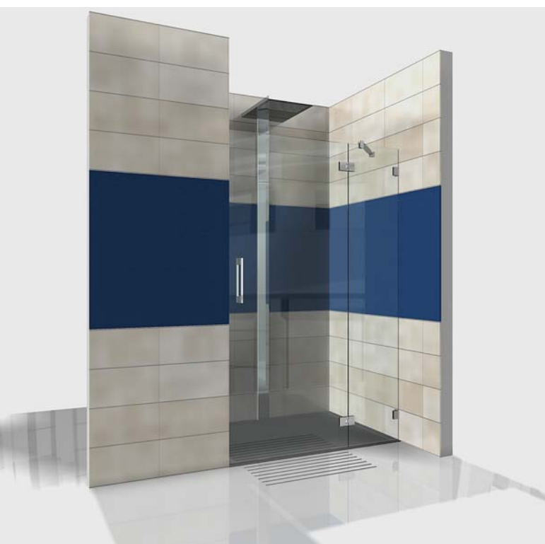
Variante 3 Nischendusche mit 1 Tür, Festteil, Griffstange, Stabilisations- stange 45°, Dichtungen und Schwallenschutz
